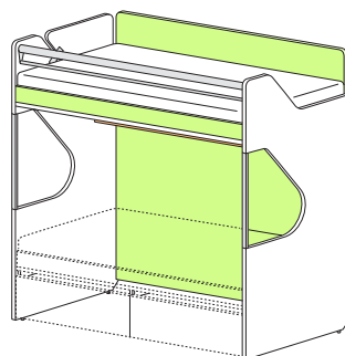
Bunk bed module
