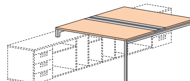
Столы письменные с откидными планками на полукаркасе
